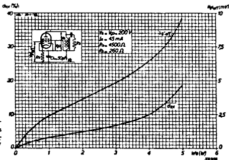
Bild 622. Klirrfaktor und notwendige Gitterwechselspannung als Funktion der Ausgangsleistung für 200 V Betriebsspannung und 9 W Einstellung.
